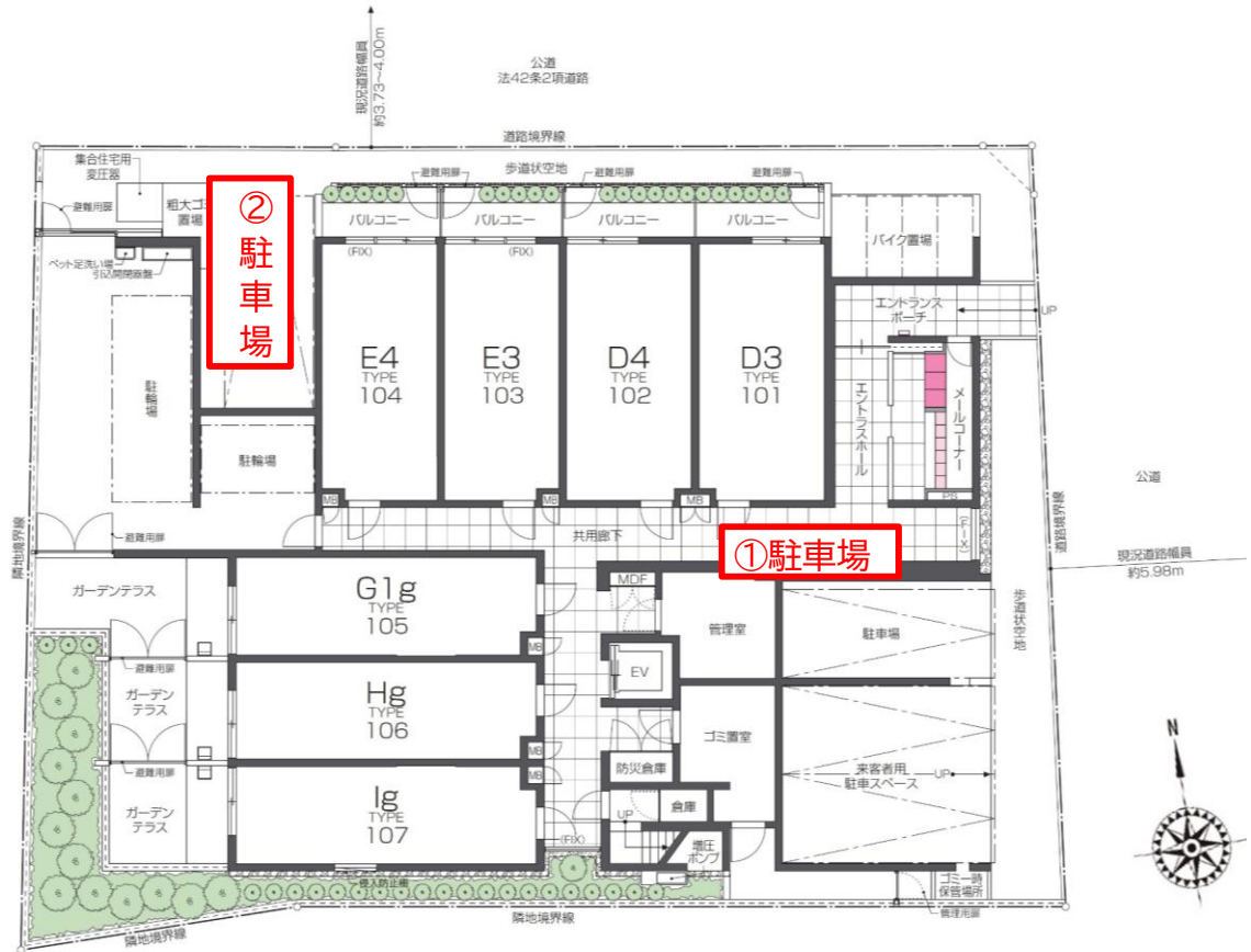
■配置図
