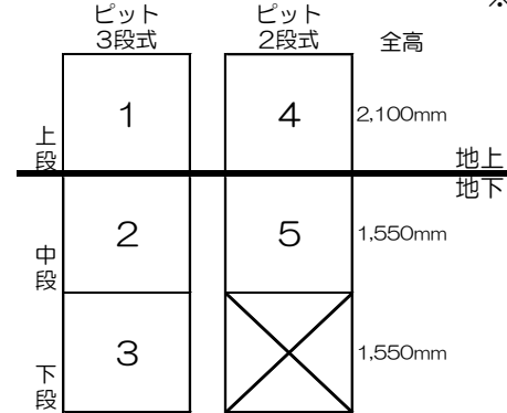
【機械式駐車場 配置図】
