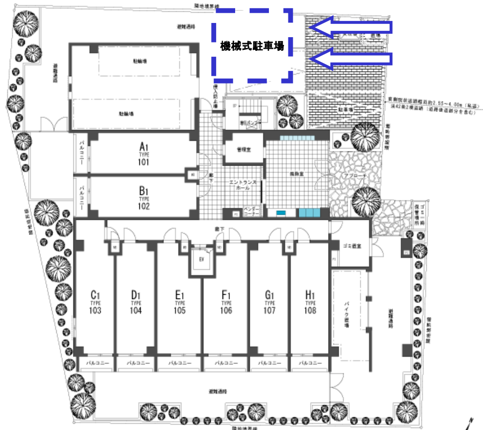
1F平面図
