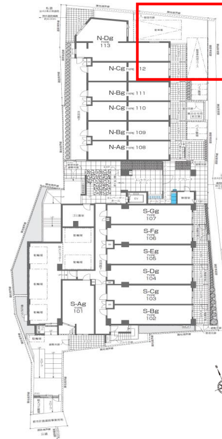
駐車場配置図
